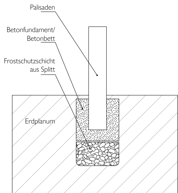
Aufbau einer Palisadeneingrenzung
